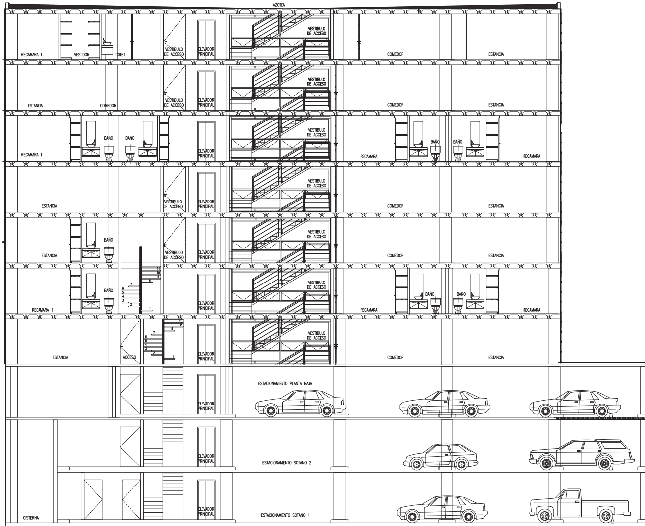
corte longitudinal
