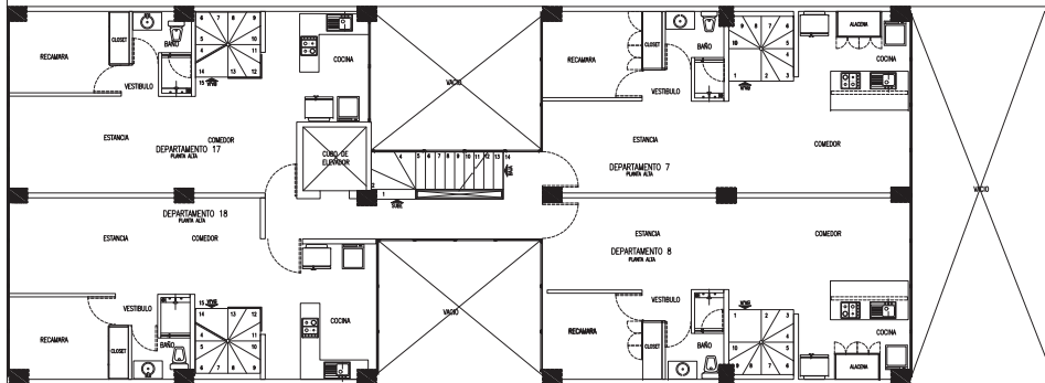
planta sexto piso
