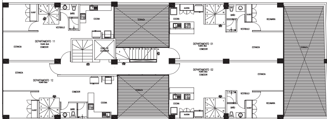
planta primer piso
