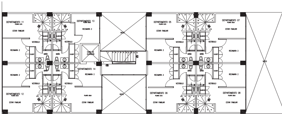
planta quinto piso
