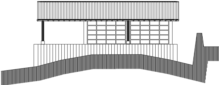
fachada lateral
