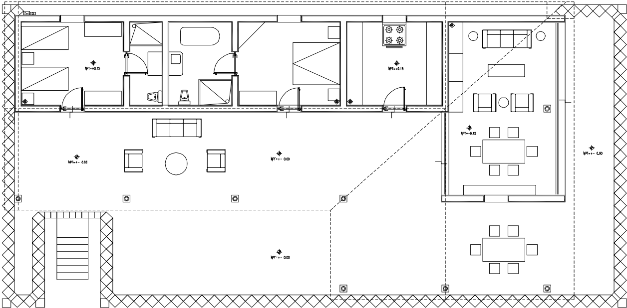
planta arquitectónica
