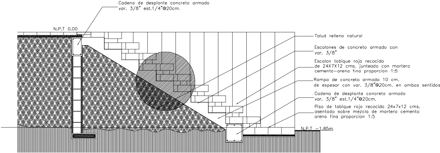
corte escalera acceso
