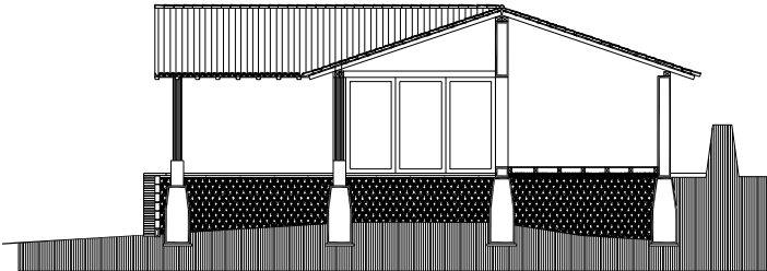
corte
